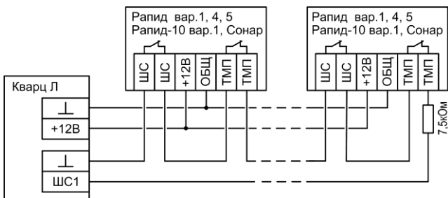
Рис.А7 Схема подключения охранных извещателей Рapid var.1,4,5, Рapid-10 var.1, СОНАР
