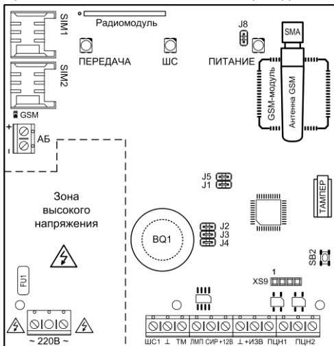
Рис.1 Плата прибора (вариант с радиомодулем)
