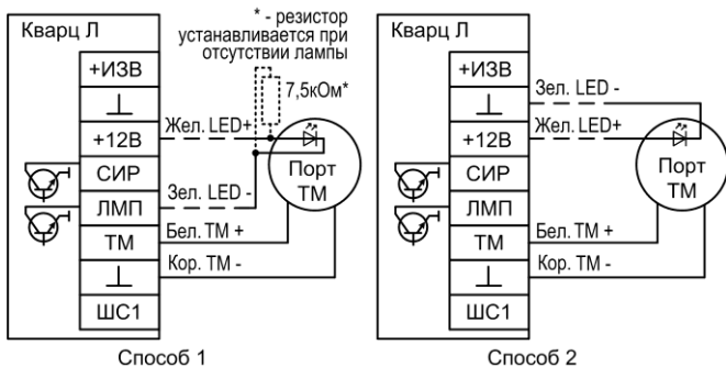
Рис.А2 Схемы подключения порта ТМ
