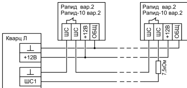
Рис.А6 Схема подключения охранных извещателей Рapid var.2, Рapid-10 var.2
